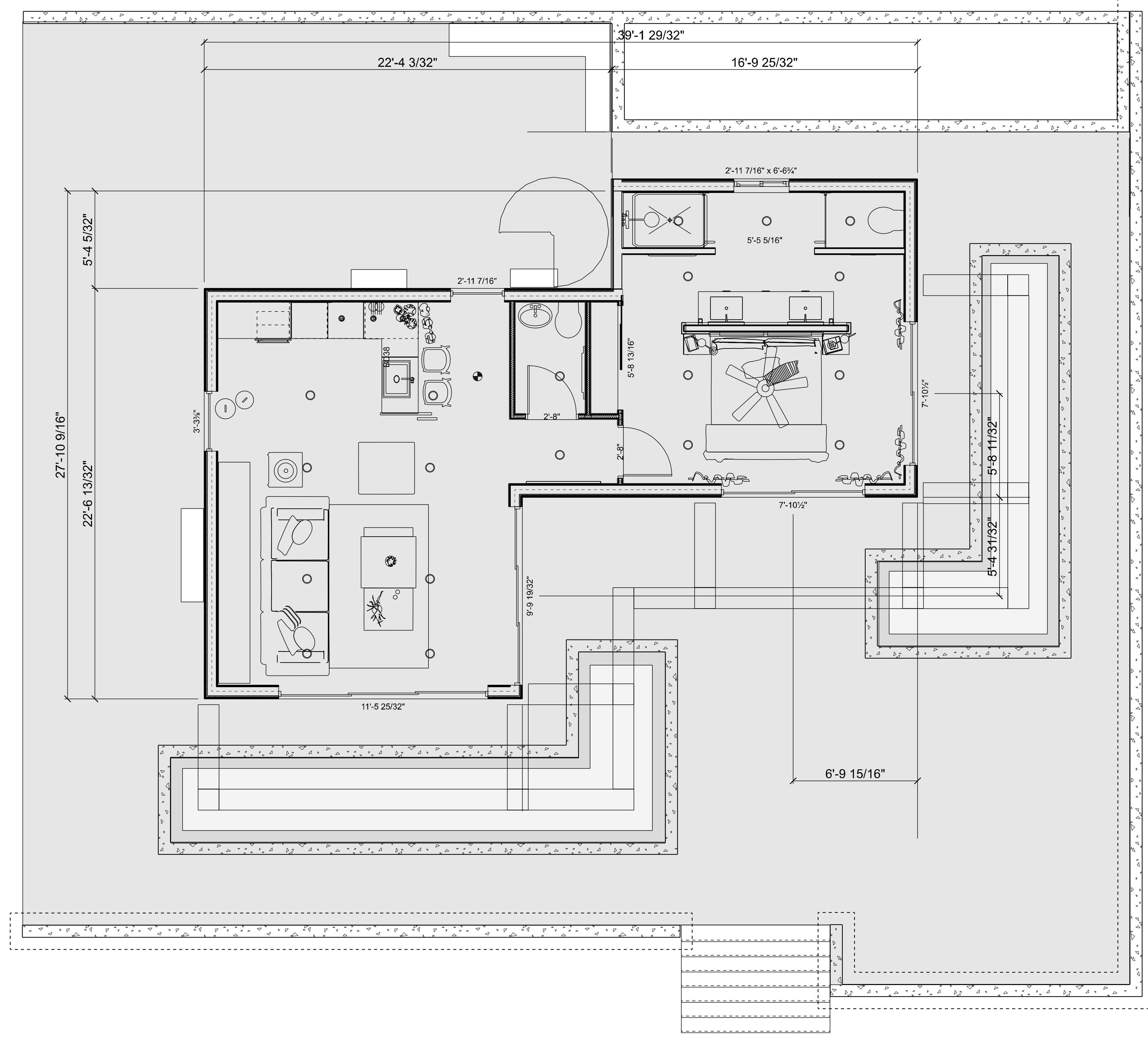
Grenada Luxe Floorplan SCALE: 0.2813" = 1'-0"
